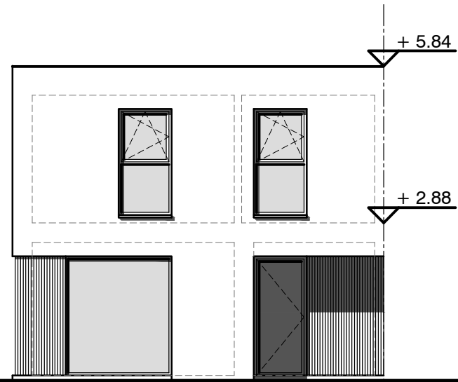
voorgevel
