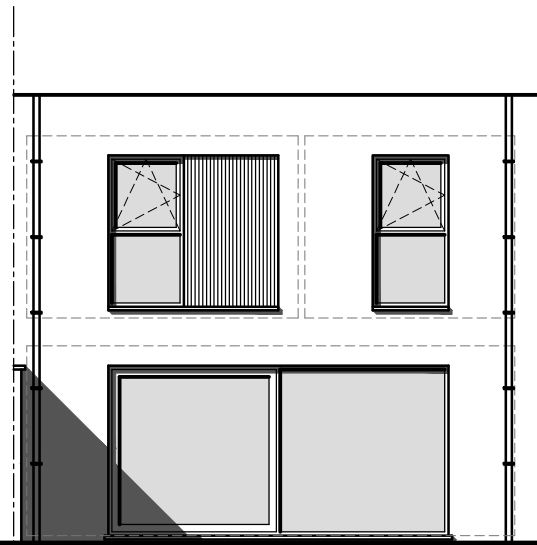
achtergevel
