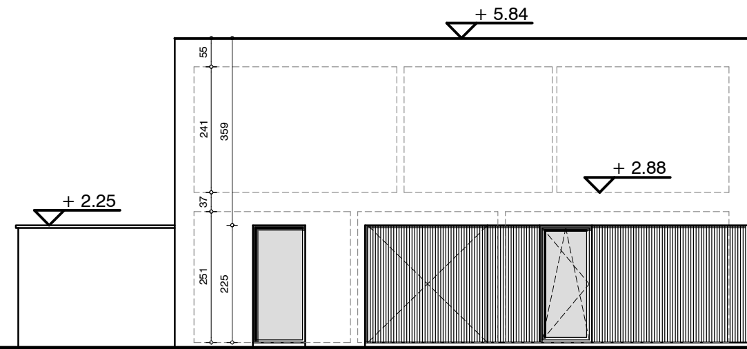
zijgevel links
