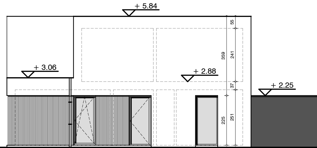
zijgevel rechts
