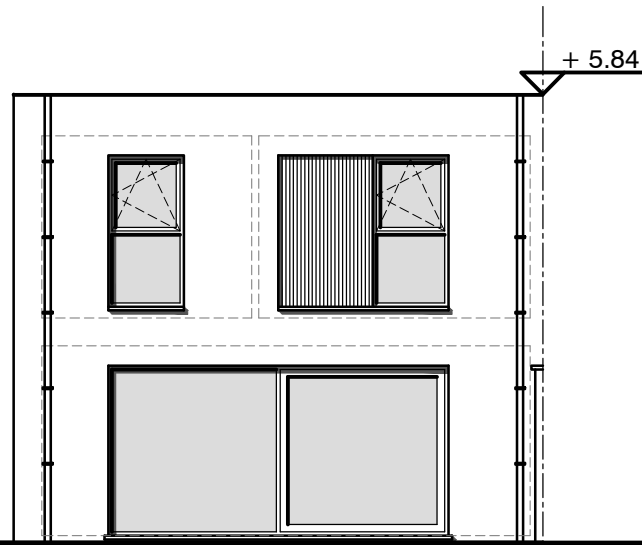
achtergevel
