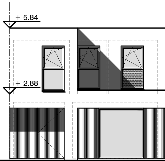
voorgevel
