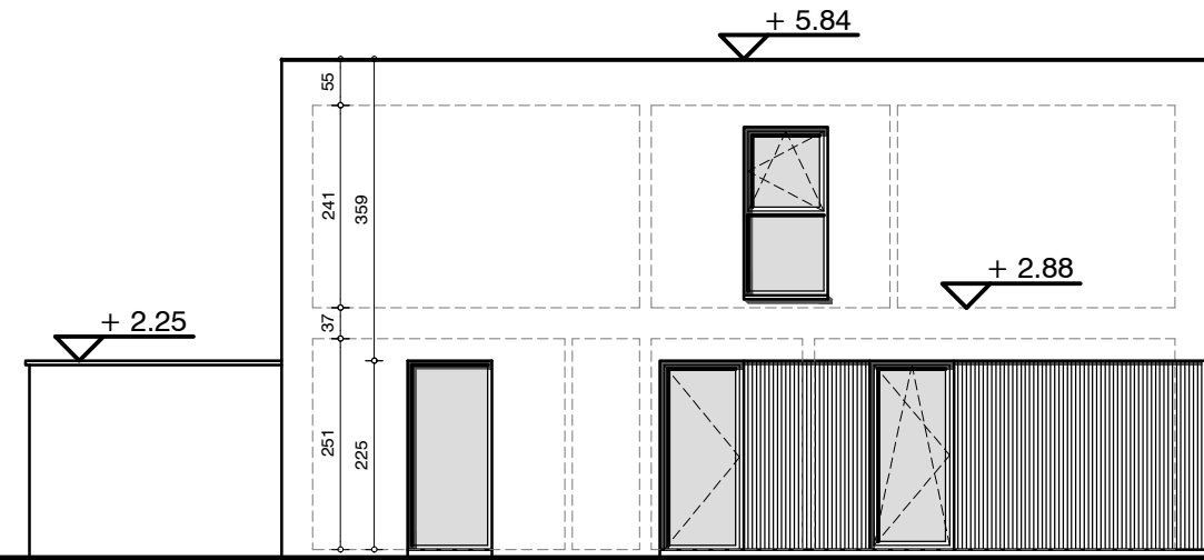
zijgevel links
